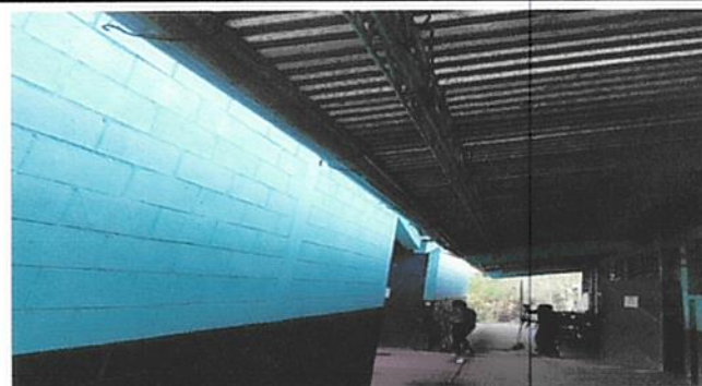
Foto 8: Sustitución de canal de metal y reparación de bajada de agua pluvial
